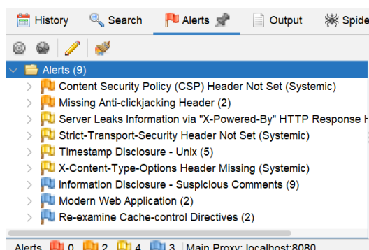
Gambar 11. Hasil Scan ZAP MAN 2 Situbondo
